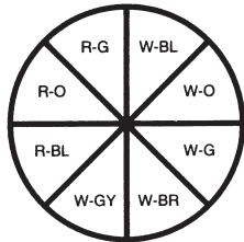
200 PAIR
